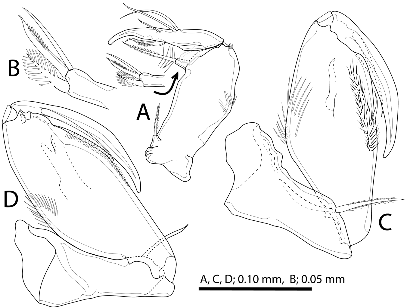
Fig. 6. Peltidium penyui , new species, female holotype (UKMMZ-1638). A, right maxilla, anterior view; B, distal endite of maxilla, anterior view; C, right maxilliped, anterior view; D, left maxilliped, posterior view.
